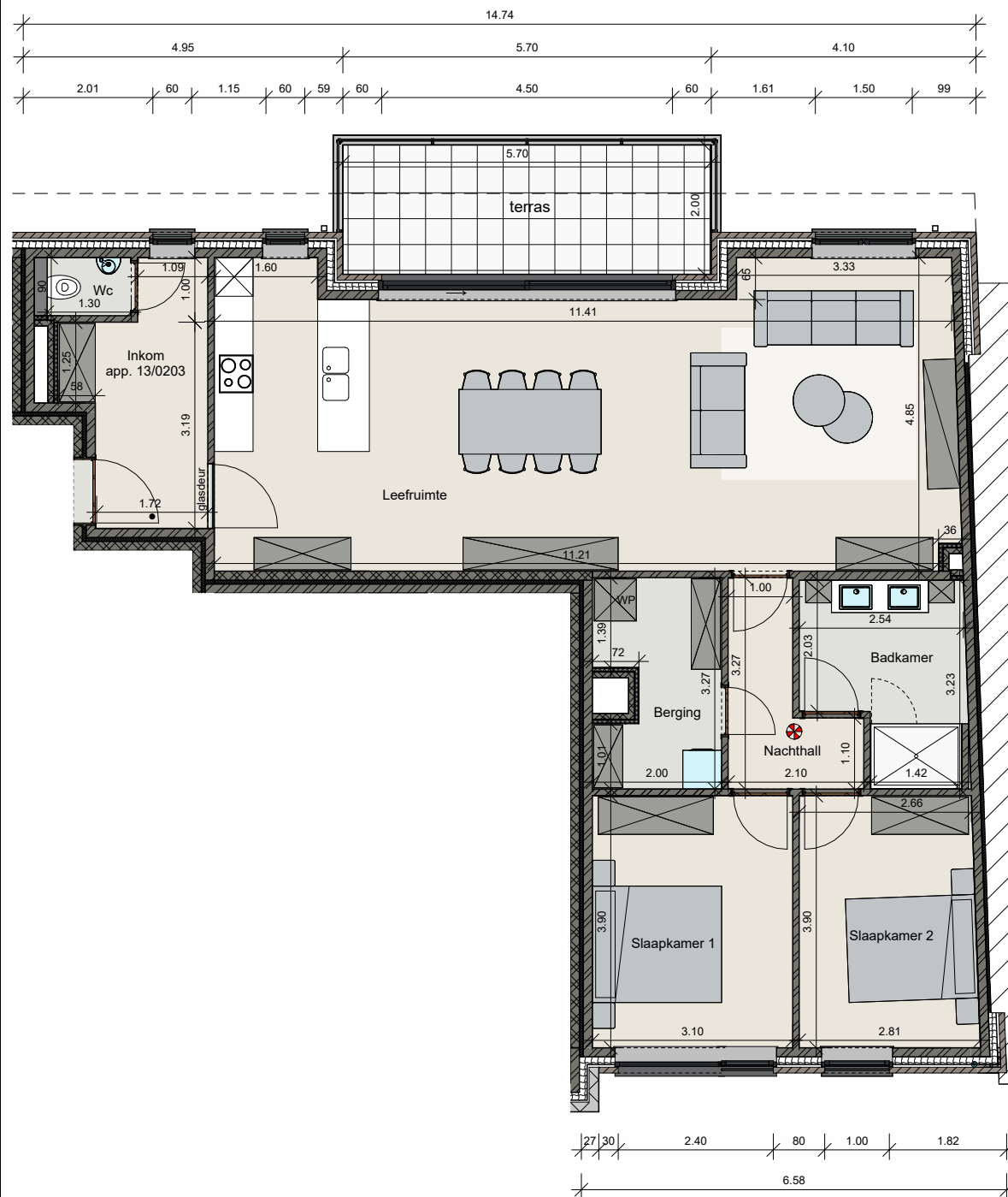
Grondplan, schaal 1/100
