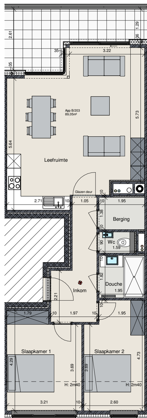
Grondplan
