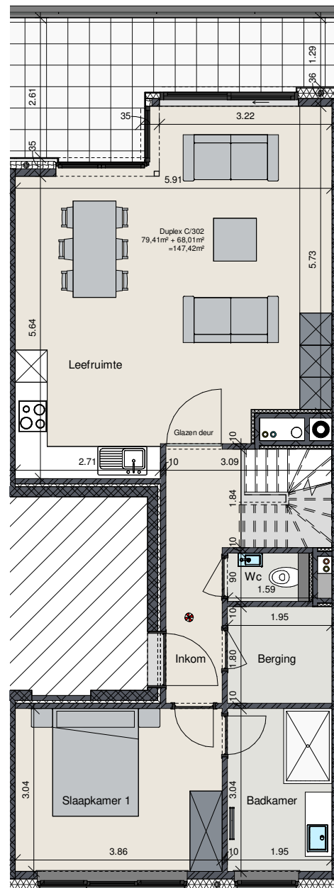
Grondplan
