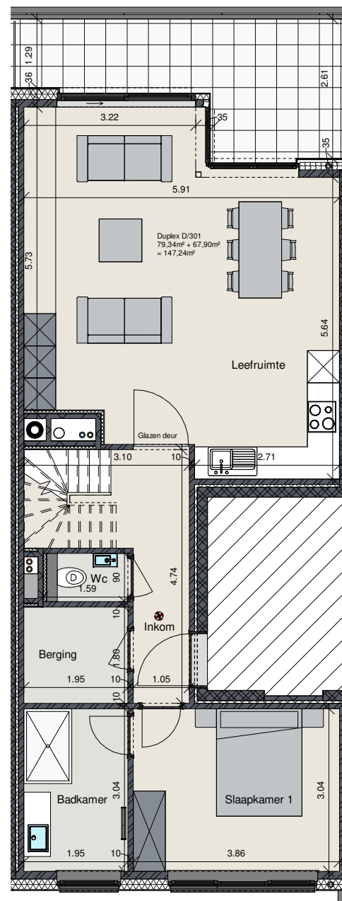
Grondplan
