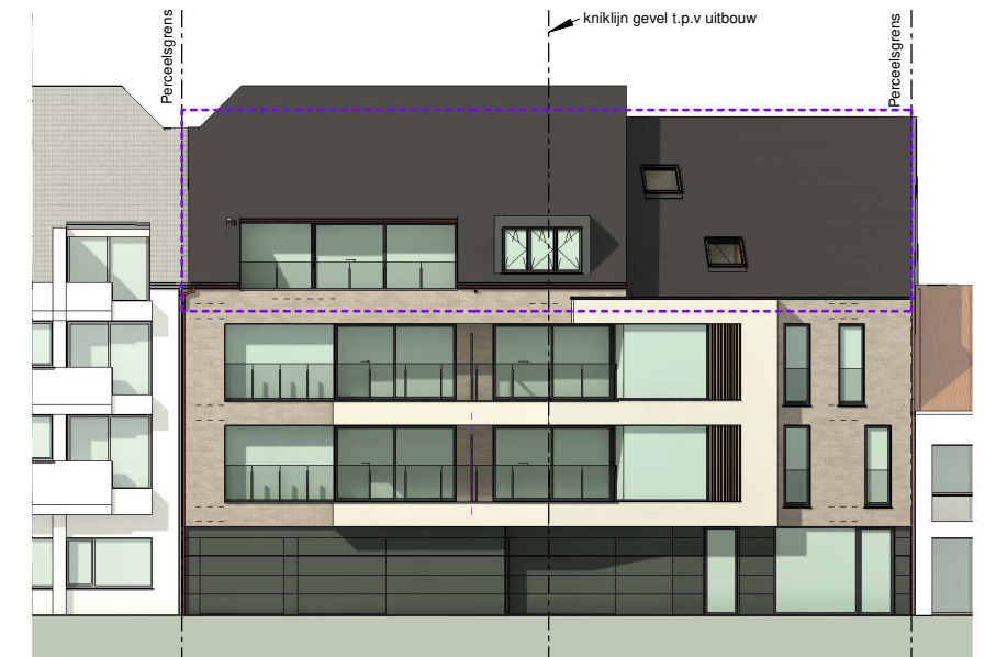
Zuidgevel
